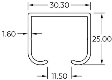
Top Track 2213 WT : 0.381 KG/M
