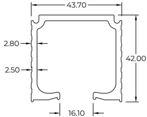
Top Track 11938 WT : 1.091 KG/M
