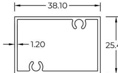
1410122 WT : 0.459 KG/M
