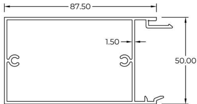
7020154(M)
