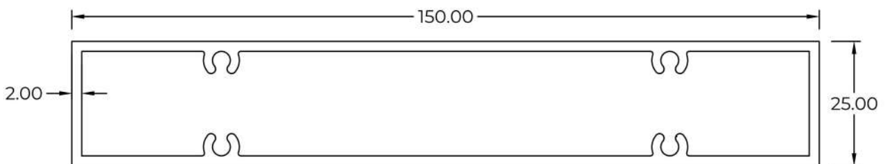
6010204(M) WT : 2.038 KG/M
