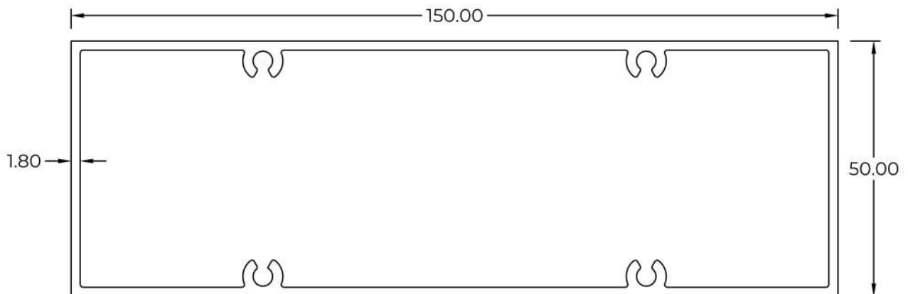
6020184(M) WT : 2.150 KG/M
