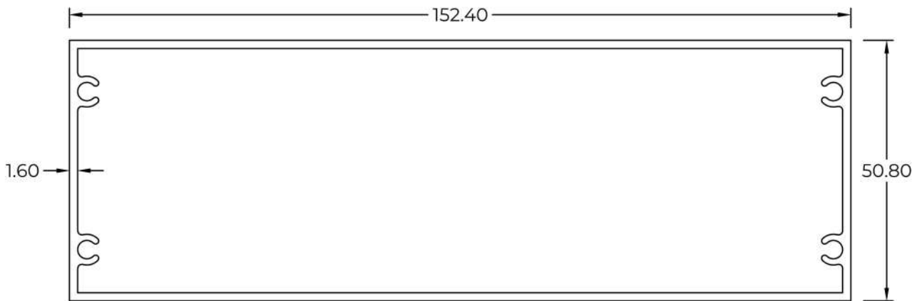
6020164 WT : 1.858KG/M
