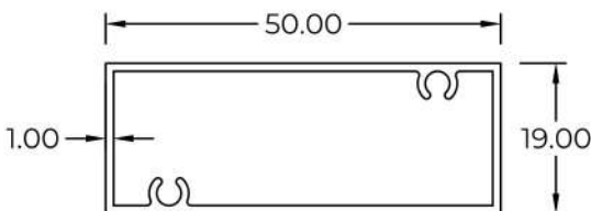
2006102(M) WT : 0.404 KG/M
