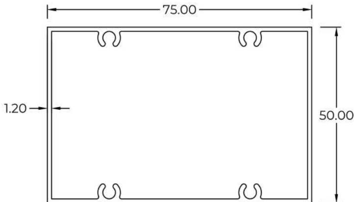
3020124(M) WT : 0.939 KG/M
