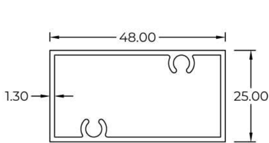
1710132(M) WT : 0.572 KG/M
