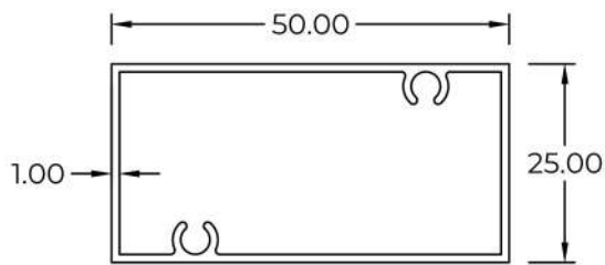
2010102(M) WT : 0.446 KG/M
