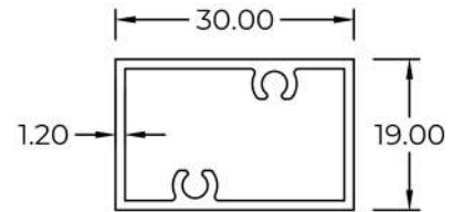
1206122(M) WT : 0.363 KG/M
