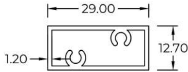
1104122 WT : 0.331 KG/M
