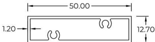
2004122 WT : 0.468 KG/M
