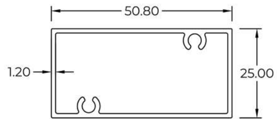
2010122 WT : 0.554 KG/M
