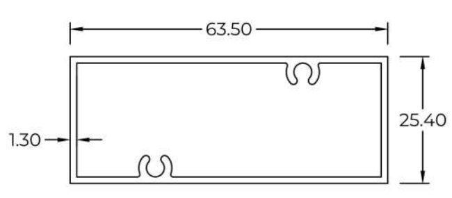
2410132 WT : 0.684 KG/M
