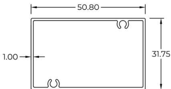
2012102 WT : 0.480 KG/M
