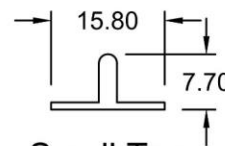
Small Tee 5904 WT : 0.086 KG/M
