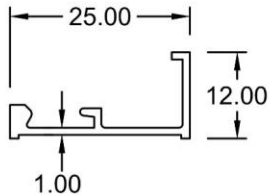
Glazing Bead SPF5 WT : 0.138 KG/M
