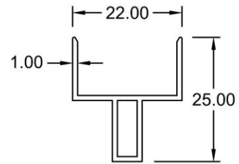
Double Glazing Adaptor 1795 WT : 0.198 KG/M
