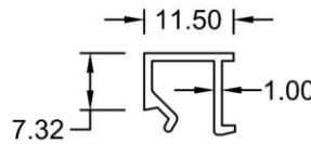
Beading SPF5A WT : 0.095 KG/M
