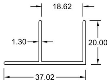
F Section 8203 WT : 0.261 KG/M
