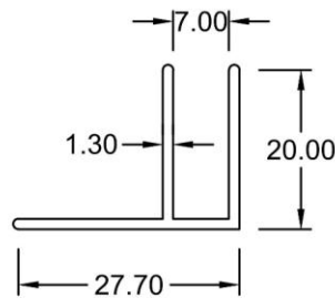
F Section 2698 WT : 0.228 KG/M
