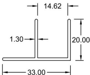
F Section 8204 WT : 0.247 KG/M
