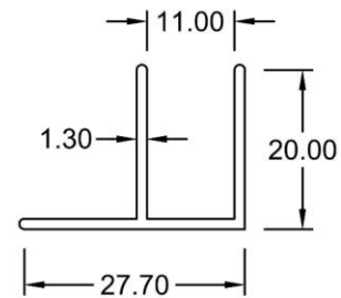
F Section 2697 WT : 0.228 KG/M
