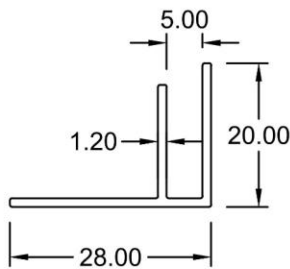
F Section 8205 WT : 0.203 KG/M
