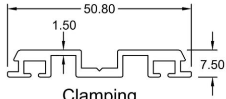
Clamping 4333 WT : 0.467 KG/M
