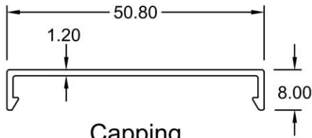
Capping 4332 WT : 0.217 KG/M
