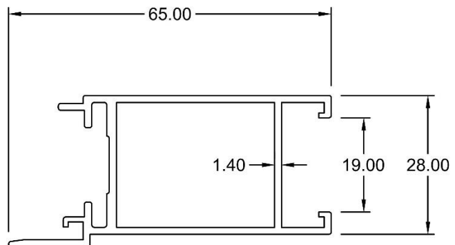
Inner w/o Hook 2111Z WT : 0.765 KG/M
