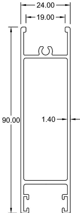
Inner Bottom 2108Z WT : 0.963 KG/M
