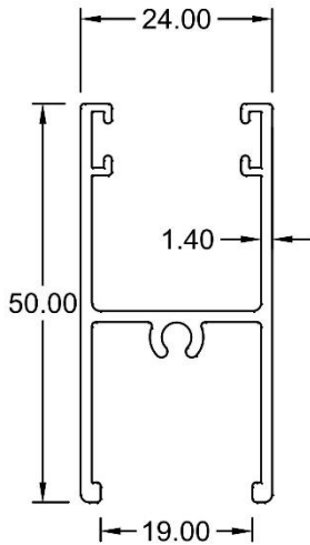
Inner Top 2107Z WT : 0.555 KG/M
