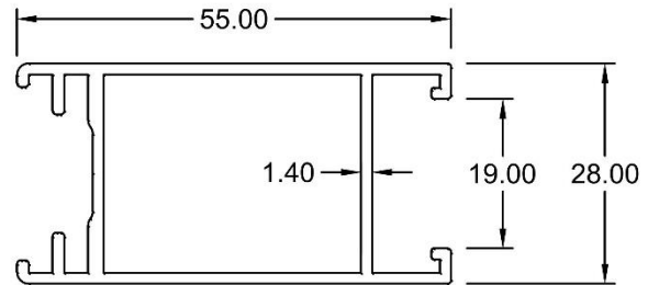
Inner 2109Z WT : 0.713 KG/M
