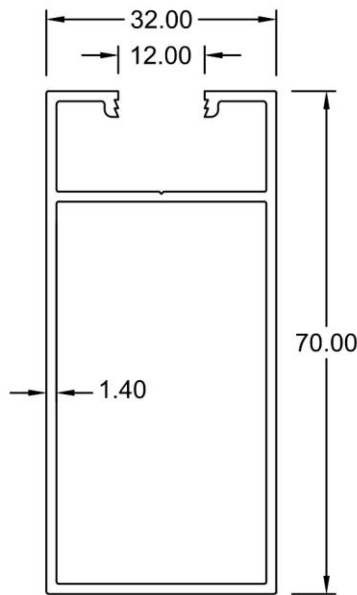
14212 WT : 0.834 KG/M
