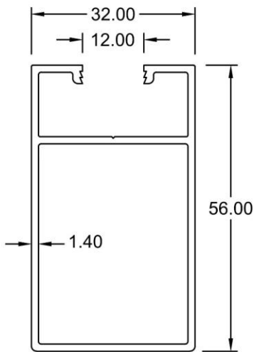
11202 WT : 0.727 KG/M
