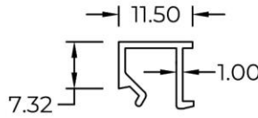
Beading SPF5A
