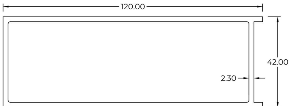
15895 WT : 1.965 KG/M
