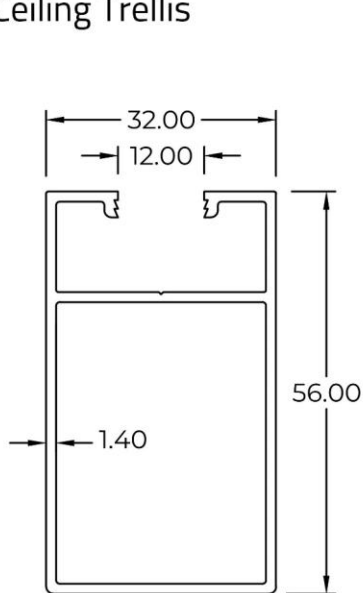
11202 WT : 0.727 KG/M
