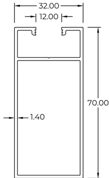
14212 WT : 0.834 KG/M
