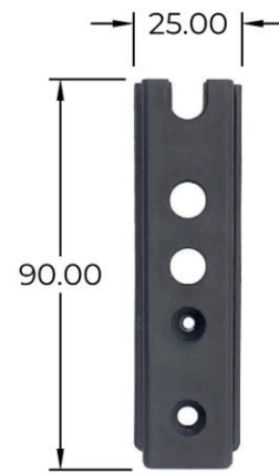
Inner Bottom Guide HDB-443 for door
